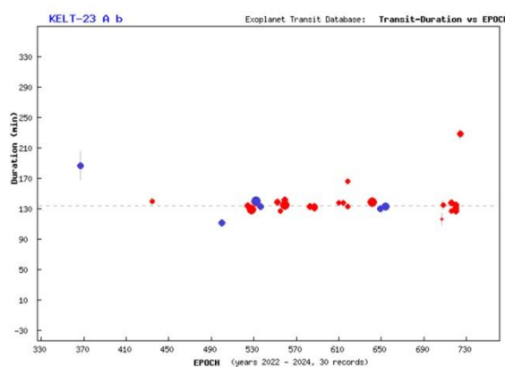
Myndir/Fig. 53a-b. a) Ljósdeyting (vegna þvergöngu), lotufföldi á þverás og bst. á lóðás. Brotalínan sýnir viðurkennda dýpt (0,0226 bst.). b) Tímalengd, lotufföldi á þverás og frávik á lóðás. Blá gildi eru mælingar höfundar. Niðurstöður fengnar af vefsvæði TRESCA. – a) Depth in mmag and b) duration of transits. Blue dots are the author's results. Data obtained from TRESCA website (Poddaný o.fl. 2010).
