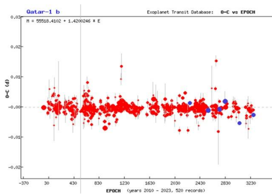
Myndir/Fig. 58a-b. a) Tímalengd þvergöngu. Fjöldi þvergöngu (lotur) á þverás en tími þvergöngu á lóðás. b) O-C rit á sama tímabili. Lotur á þverás (tímaás) með tímafrávik á lóðás. Blá gildi eru mælingar höfundar. — a) Duration of transits and b) O-C determination. Blue points are the author's results. Results based on TRESKA website (Poddaný and others 2010).
