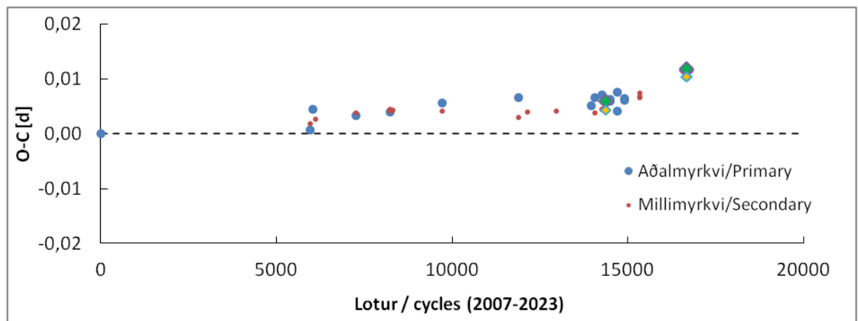
Mynd 18. Rauntíma mínus spátíma rit (O—C rit) af aðalmyrkvum V 473 Cam á tímabilinu 2007-2023. Mælingar höfundar eru táknðar með grænum og gulum tíglum. Á þverás er fjöldi lotna frá því að mælingar hófust en þar vísar „núll“ á viðmiðstíma sem B.R.N.O. notar. Á lóðás stendur „núll“ fyrir spátíma reglulegrar birtulotu. Gögn í O—C ritið eru fengin frá vefsetri B.R.N.O. (2025) en myndin var aðlöguð að þessari samantekt. — The O—C diagram contains HJD timings of primary (blue dots) and secondary (red dots) eclipses, observed between 1926 and 2023. Data in the O—C plot were obtained from the B.R.N.O. website (2025), but the image was adapted for this compilation. The number of cycles is plotted on the x-axis and time deviation, based on the B.R.N.O. Epoch, on the y-axis. The author's measurements are represented by green and yellow diamonds.
