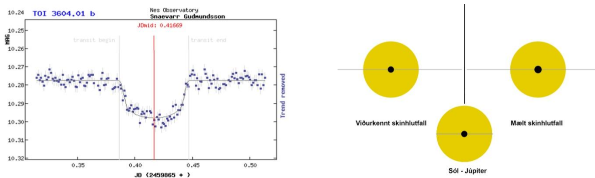
Myndir/Fig. 25a-b. a) Birtugildi í þvergöngunni 12. október 2022. b) Skinhlutfall. Niðurstöðurnar lýsa reikistjörnu með ~34% stærri geisla en uppgið gildi í veftóli TRESKA. – a) Results from October 12, 2022. b) Geometry as a results of measurements. Images based on TRESKA website (Poddaný and others 2010).
