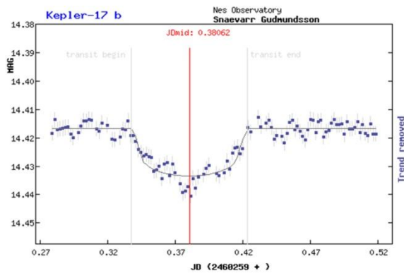
Myndir/Fig. 61a-b. a) Mæld birtugildi Kepler-17 þann 10. nóvember 2023. Tími er á þverás og birta á lóðás. b) Dýpt þvergöngu samkv. TRESKA. Brotalínan sýnir viðurkennda dýpt (0.0213 bst.). Blátt gildi er mæling höfundar. Niðurstöður fengnar á vefsvæði TRESKA. — a) Results from November 10, 2023. Time is on the x-axis and magnitude on the y-axis. b) Transit depth comparison. Results obtained from the website of TRESKA (Poddaný and others 2010).
