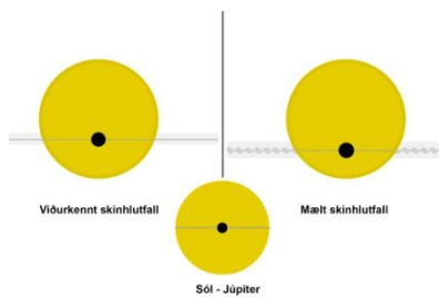
Myndir/Fig. 34a-b. Skinhlutfall, ráðið af birtuferli. Niðurstöður t.v. a) 12. janúar benda til reikistjörnu með ~8% stærri geisla og ~3% meiri brautarhalla, og t.h. b) 17. desember, 2023, ~6% stærri geisla og ~0,7% minni brautarhalla en viðurkennd gildi. — Geometry derived from the measurements. Results from a) January 12, and b) December 17, 2023. Image based on TRESCA website (Poddaný and others 2010).
