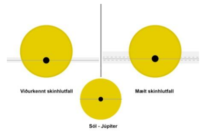
Myndir/Fig. 34a-b. Skinhlutfall, ráðið af birtuferli. Niðurstöður t.v. a) 12. janúar benda til reikistjörnu með ~8% stærri geisla og ~3% meiri brautarhalla, og t.h. b) 17. desember, 2023, ~6% stærri geisla og ~0,7% minni brautarhalla en viðurkennd gildi. — Geometry derived from the measurements. Results from a) January 12, and b) December 17, 2023. Image based on TRESCA website (Poddaný and others 2010).
