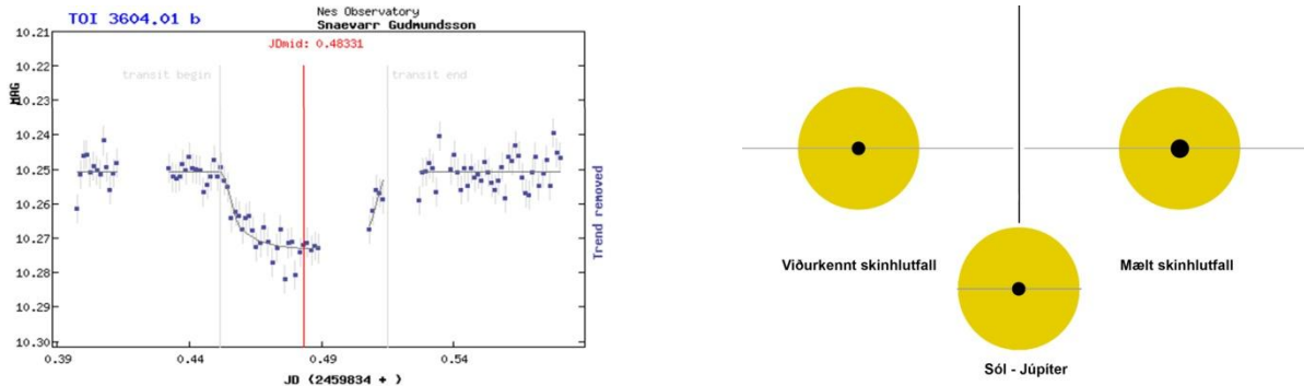
Myndir/Fig. 24a-b. a) Birtugildi TOI 3604 í þvergöngunni 11. september 2022. b) Skinhlutfall. Niðurstöðurnar lýsa reikistjörnu með ~39% stærri geisla en uppgið gildi í veftóli TRESKA. – a) Results from September 11, 2022. b) Geometry as a results of measurements. Images based on TRESKA website (Poddaný and others 2010).
